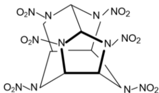
Hexanitrohexaazaisowurtzitane, (CL-20)
